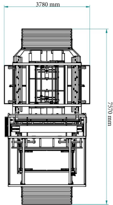
Footprint Makina Yerleşim
