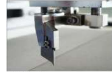
切刀装置
