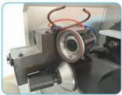
修刀裝置 Tool trimmer
